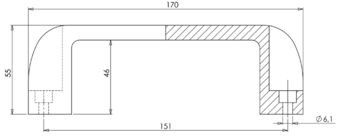
KESİT A-A
